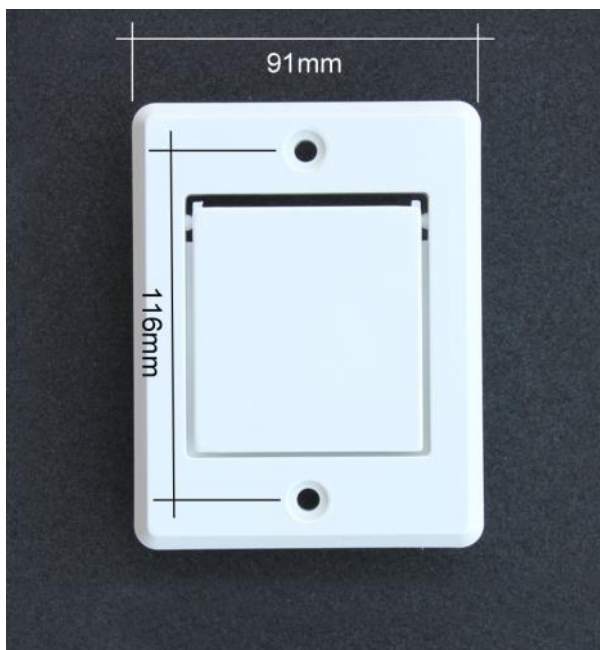
ID-52: Måttuppgifter sett framifrån.
