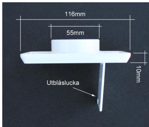
ID-52: Måttuppgifter sett från sidan.
